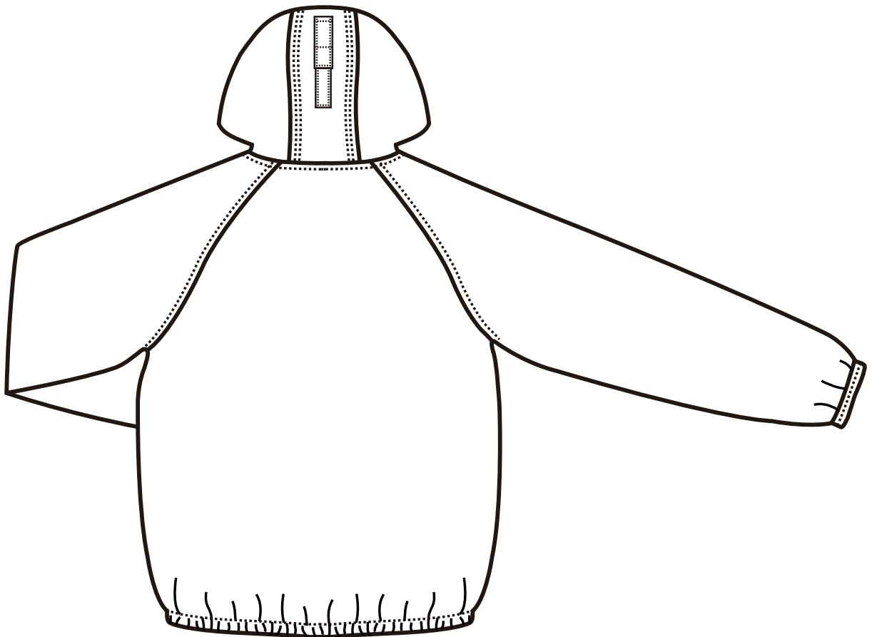
后幅
